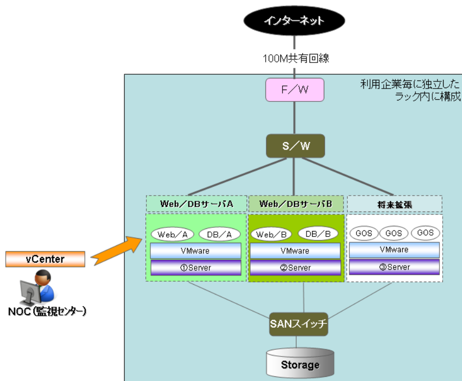
【図1】「プライベートクラウド」構成例のイメージ (VMWare で構築した場合)
