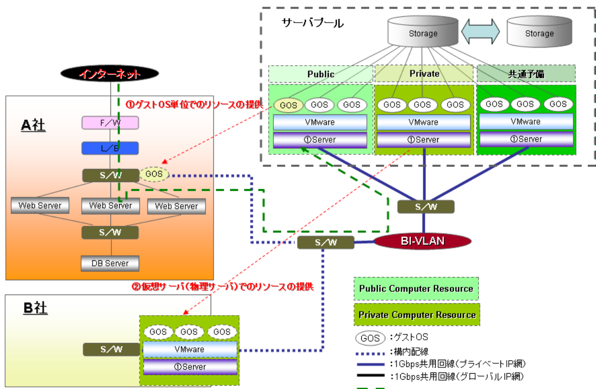
【図】「サーバオンデマンド」構成概要
